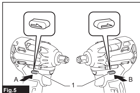
Fig. 5 ► 1. Palanca del interruptor de inversión
